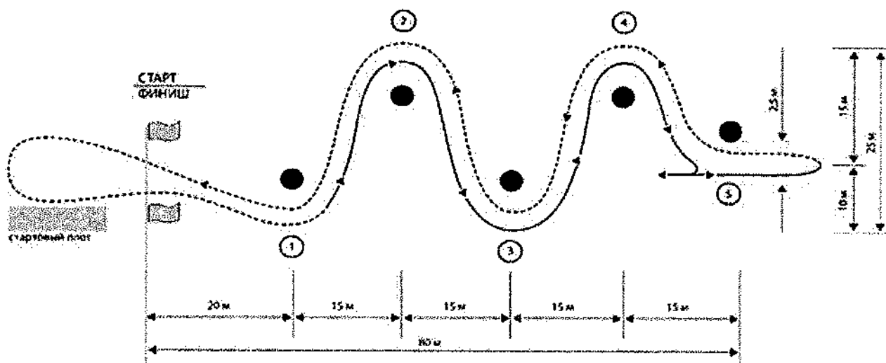
Схема трассы КЛАСС 2
