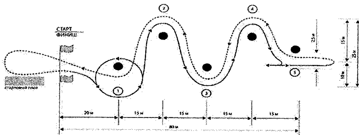
Схема трассы КЛАСС 3
