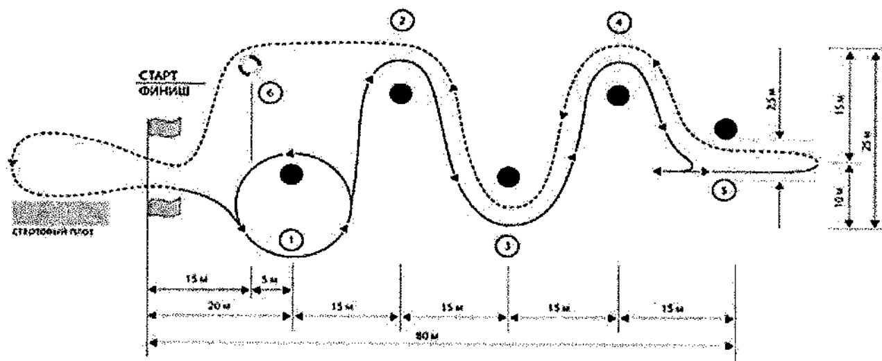
Схема трассы КЛАСС 4
