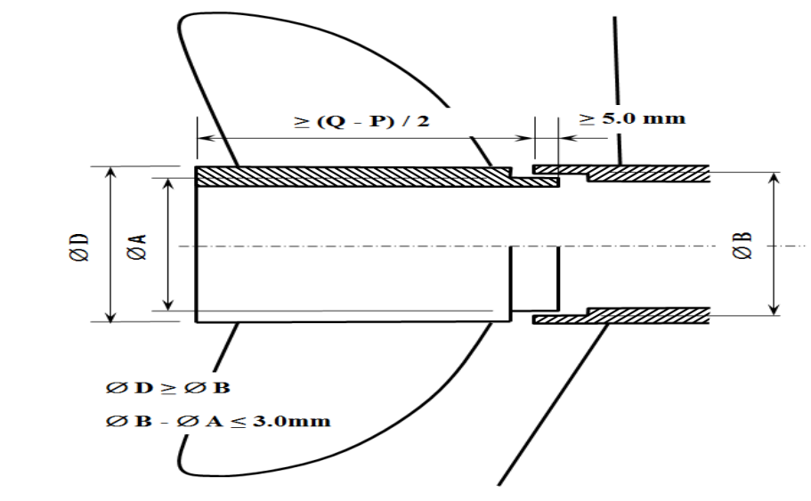
Рисунок 14. Винт
