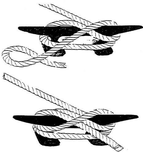
швартовочный узел
