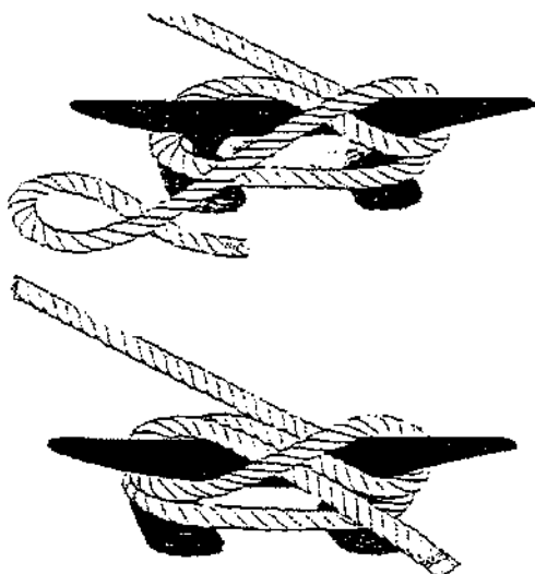
швартовочный узел
