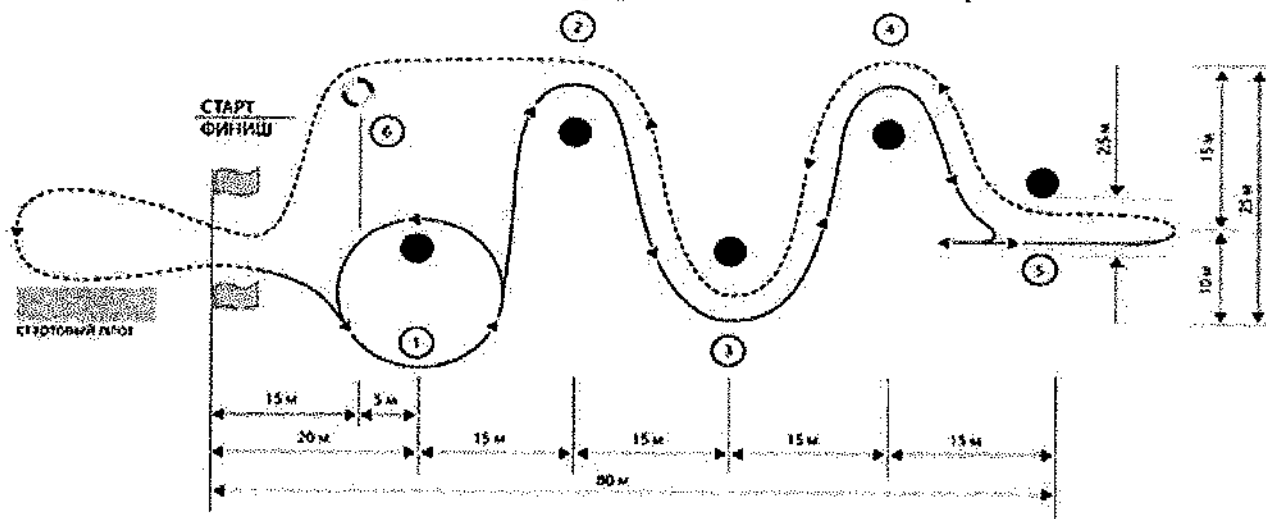
Схема трассы скоростного маневрирования класс 4 Схема трассы КЛАСС 4
