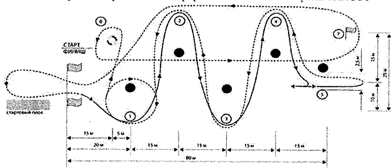
Схема трассы скоростного маневрирования класс 5 Схема трассы КЛАСС 5
